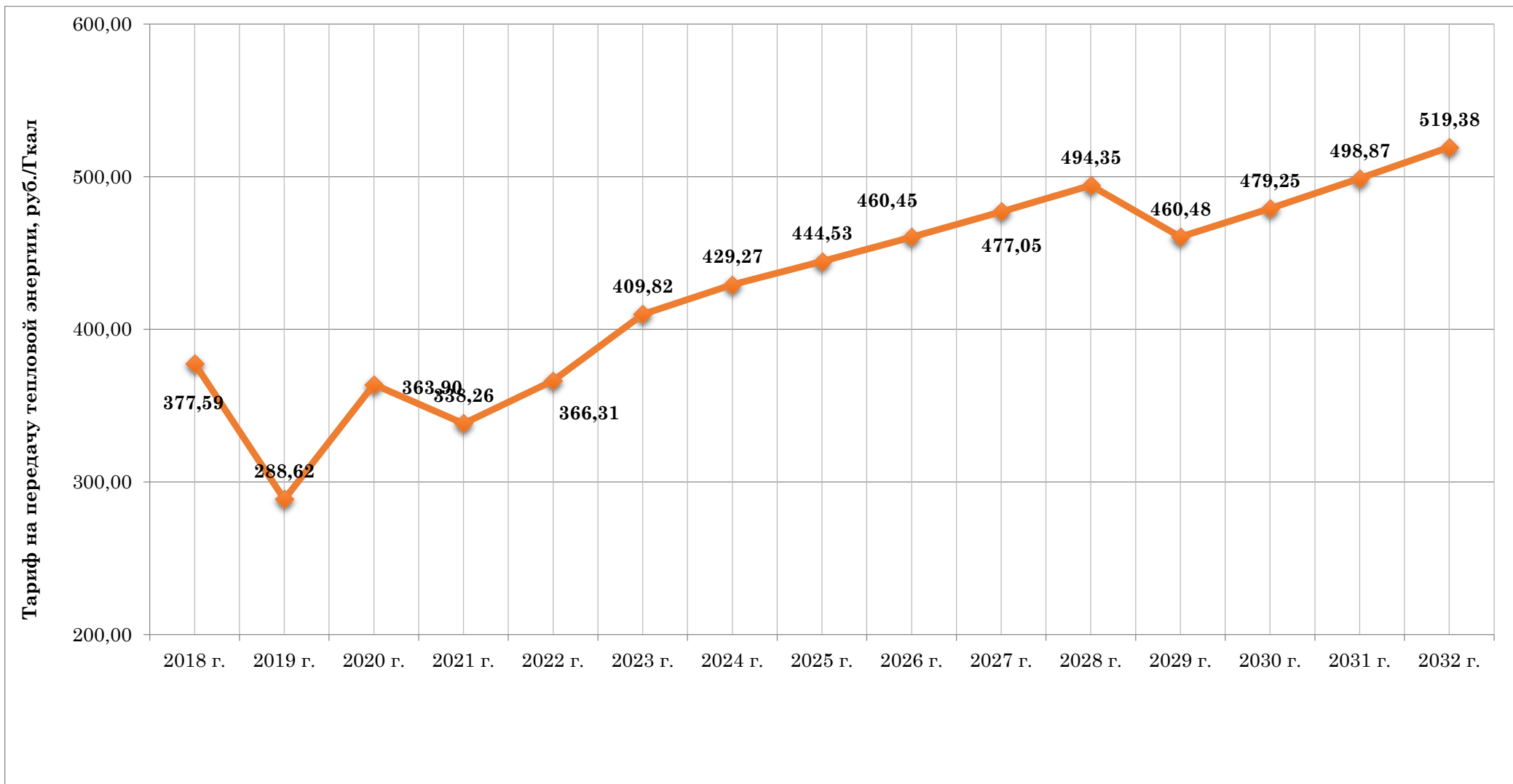
Диаграмма 1.2 – Динамика конечного тарифа конечного тарифа на передачу тепловой энергии МУП «Водоканал-Ревда» в системе теплоснабжения котельной на ул. Умбозерская, д.6 в зоне деятельности единой теплоснабжающей организации АО «МЭС» с учетом предложений по реконструкции, модернизации тепловых сетей на период до 2032 года
